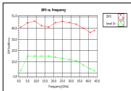
IIP3
