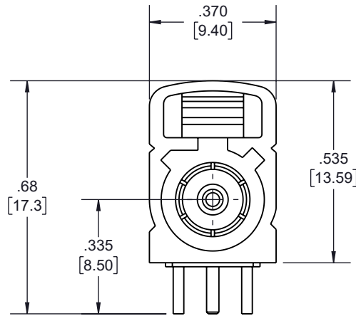
FAKRA JACK RA A CODING BLACK
